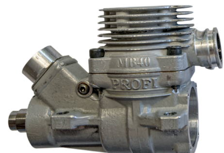
Le bloc moteur composé du carter et du cylindre
